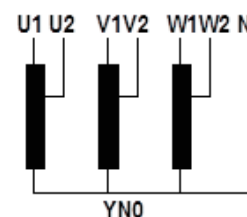
Fig.2: Elektrisch Schema
